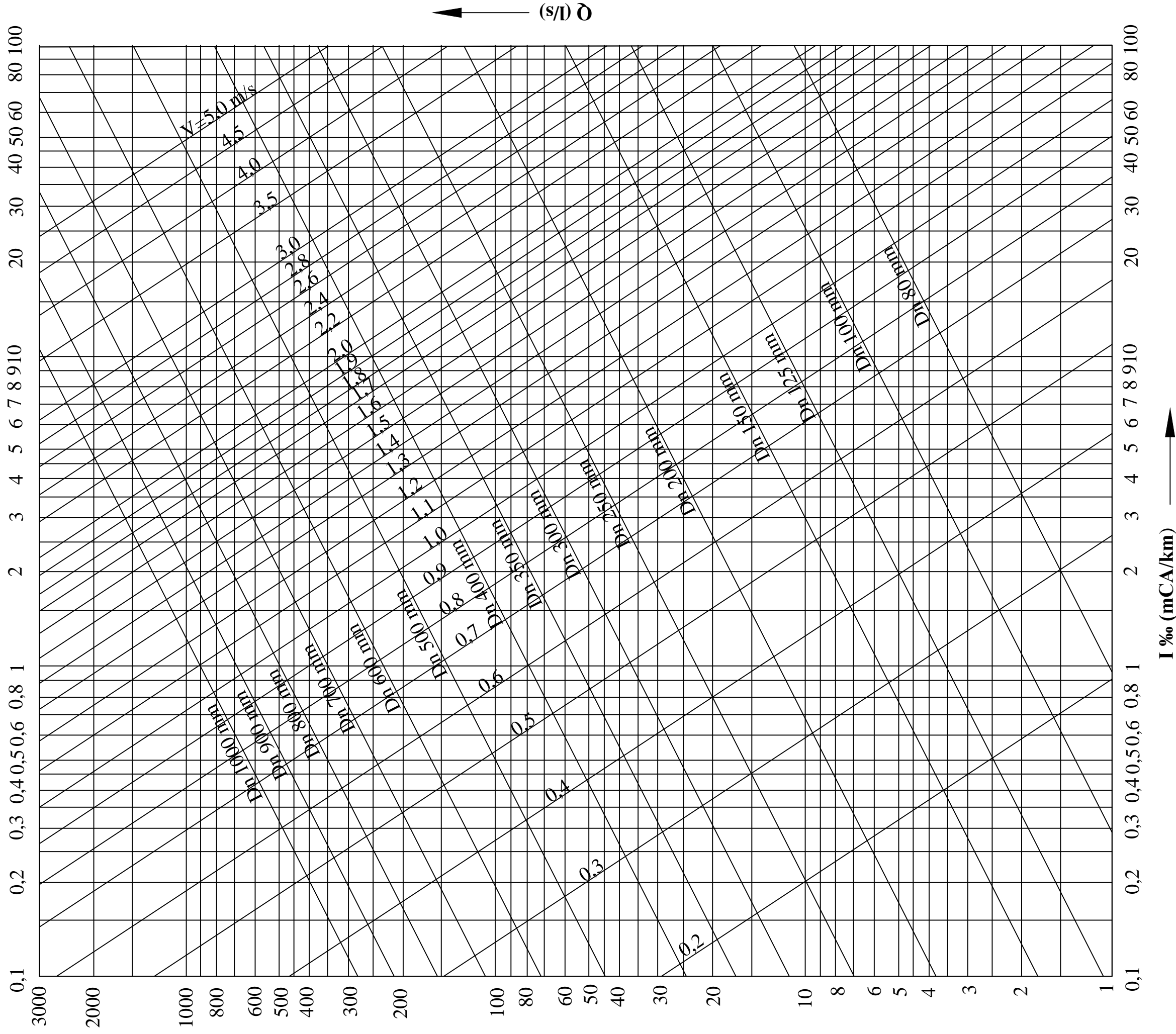
DIAGRAMA PENTRU CALCULUL CONDUCTELOR DIN PEHD
